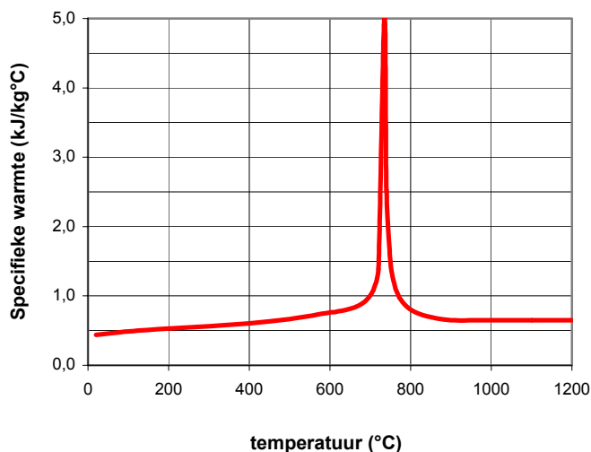
Figuur : Specifieke warmte van koolstofstaal in functie van de temperatuur [112]
