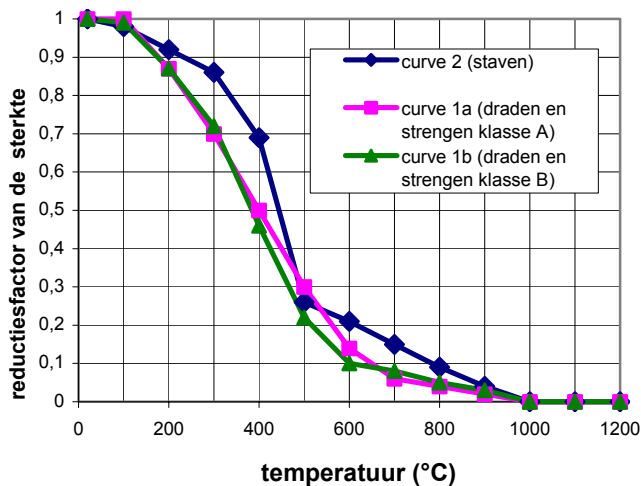
Figuur : Reductiefactor k_p(\theta) van de karakteristieke sterkte ( \beta_{f_{pk}} ) van voorspanstaal [107]
